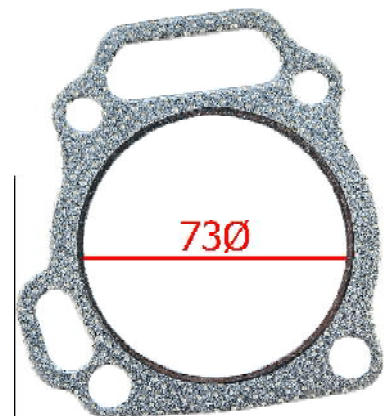
JUNTA CULATA GROSOR 1,6mm
