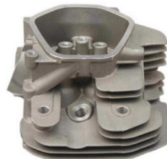
CULATA COMPLETA OHV
