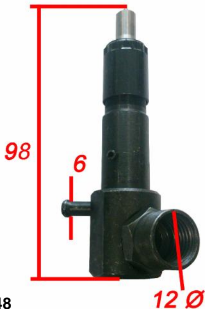
INYECTOR 186F/LA100, LA-90, LA-75
