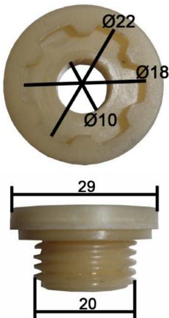
PIÑON BOMBA ENGRASE MOTOSIERRA 25 CC.
