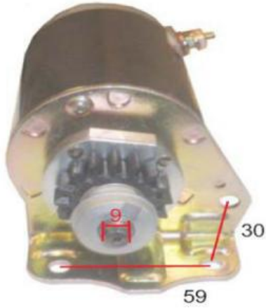
MOTOR DE ARRANQUE B&S 16Z
