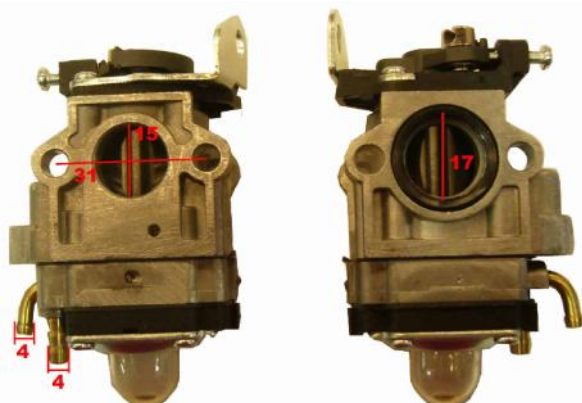
DESBROZADORA 0408520
