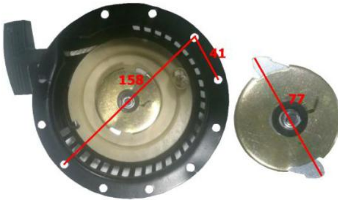
ARRANQUE COMPL. 170F/LA48/LA-40 2 PATILLAS
