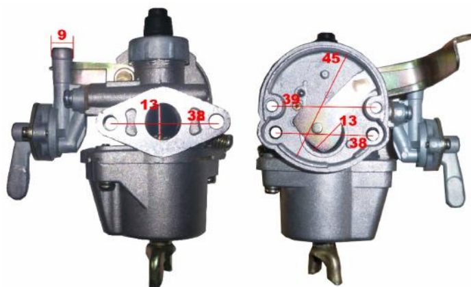
CARBURADOR DESBROZADORA 49cc
