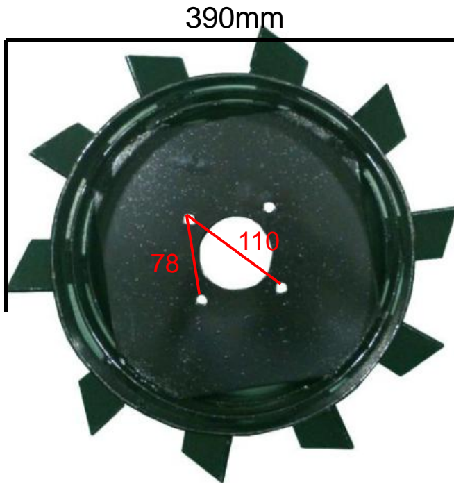
401778 JUEGO RUEDAS METALICA 4.00-8
