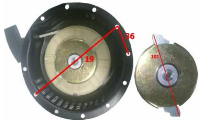
ARRANQUE COMPL. 178F/LA70/LA-60 2 PATILLAS
