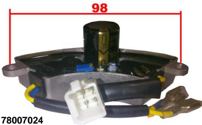
AVR MEDIA LUNA GEN 6500. 250V 470mF.
