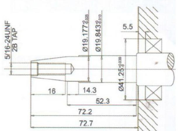
OHV200 CHAVETA V
