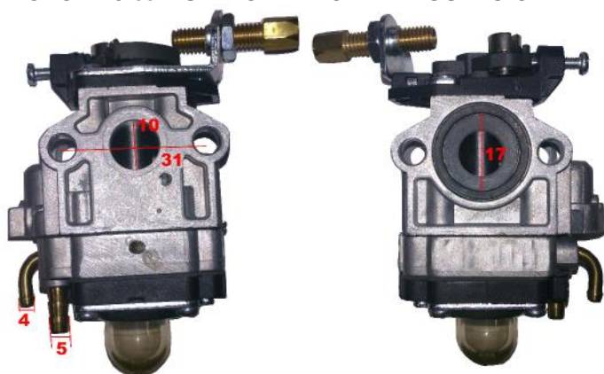
MOTOR 25 cc SIN TORNILLO DE REGULACION
