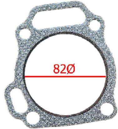
JUNTA CULATA GROSOR 1,6mm
