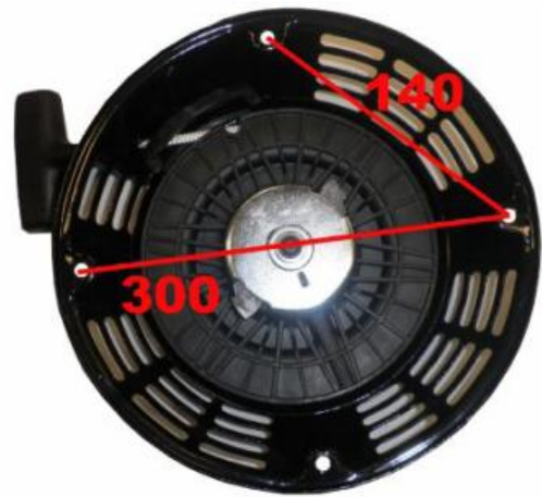
ARRANQUE LOMBARDINI 3LD 6LD 15LD
