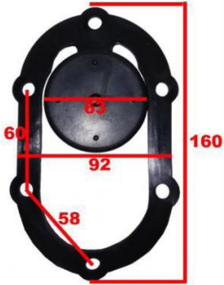
JUNTA VALVULA ASPIRACION MTB-50P
