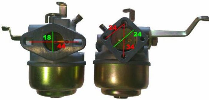
CARBURADOR ROBIN EC10
