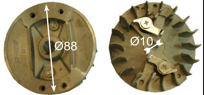
VOLANTE DE ARRANQUE 25cc
