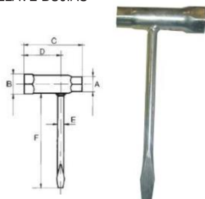
LLAVE BUJIAS
