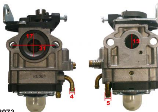
CARBURADOR COMPLETO SOPLADOR 63.3 cc Y MOTOR 51 cc
