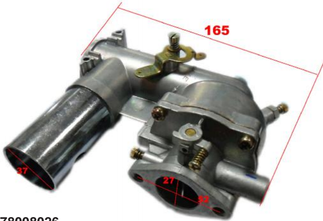
CARBURADOR B&S CPL G3
