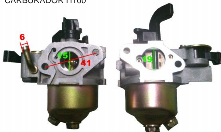
CARBURADOR H100
