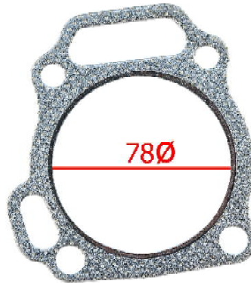
JUNTA CULATA GROSOR 1,3mm
