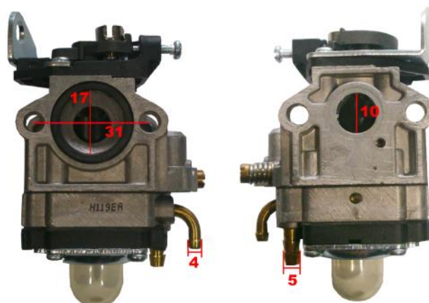
MOTOR 25cc CON TORNILLO REGULACION
