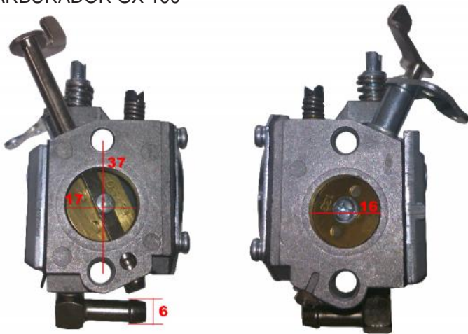
CARBURADOR GX 100
