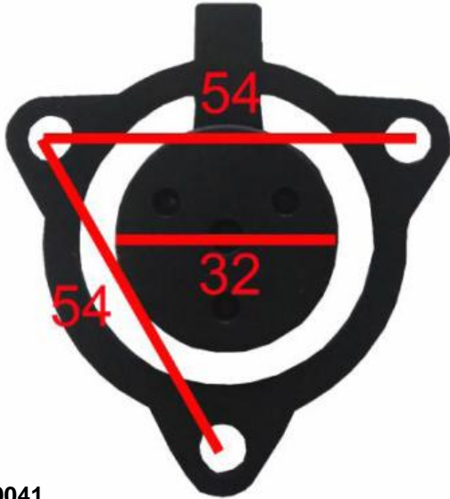
JUNTA VALVULA ASPIRACION MTB-38P
