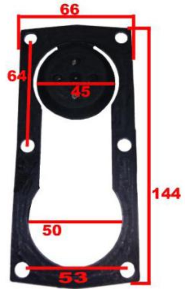
JUNTA VALVULA ASPIRACION MTB-40 TIPO W
