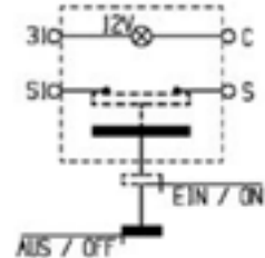
SISTEMA ELECTRICO 5
