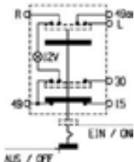
SISTEMA ELECTRICO 4
