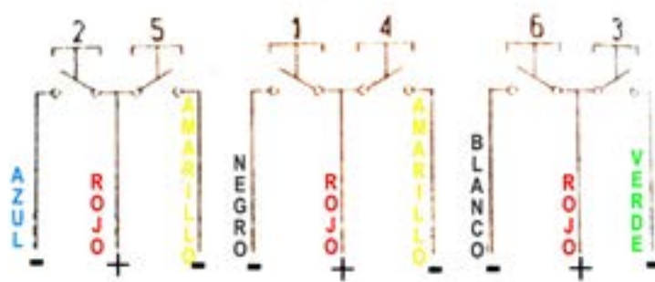
ESQUEMA ELECTRICO 6 PULSADORES
