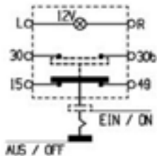
SISTEMA ELECTRICO 5
