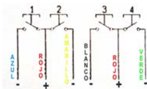
ESQUEMA ELECTRICO 4 PULSADORES
